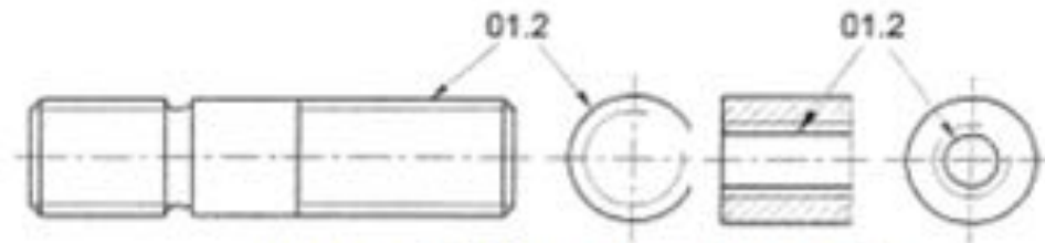
Creste di filettature (01.2.3)
